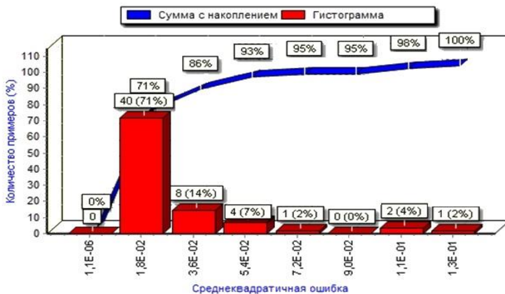
Рисунок 2. – Гистограмма распределения ошибок при обучении ИНС рисунка 1
